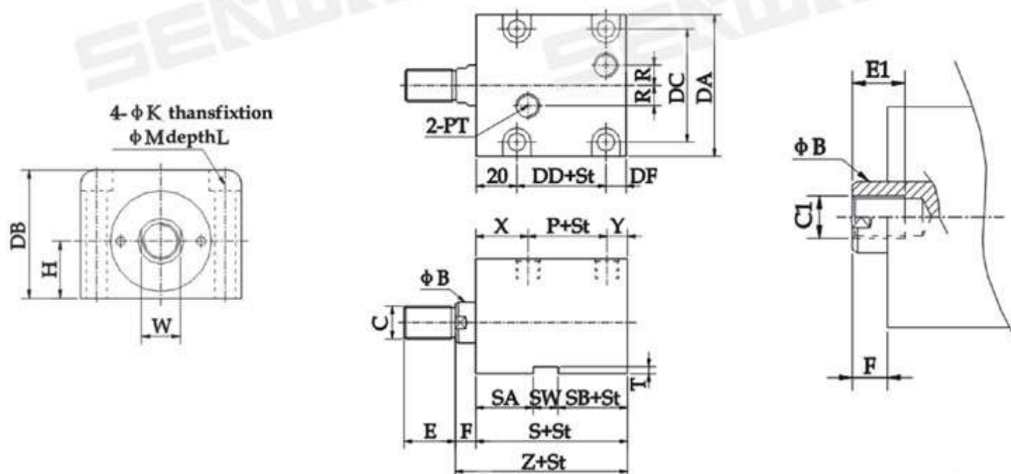
ILA 标准型 尺寸图 Standard Dimension
