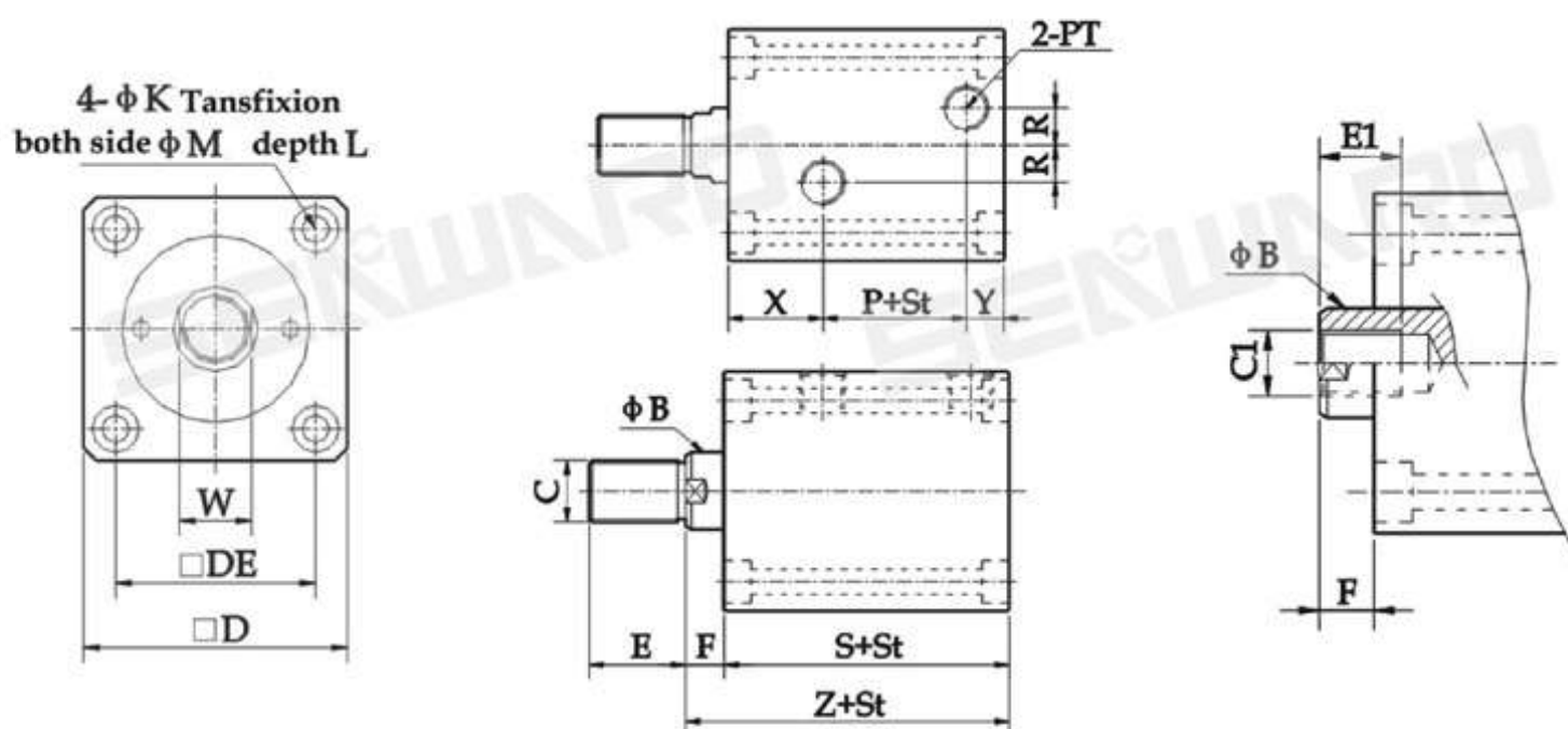
ISD 标准型 尺寸图 Standard Dimension
